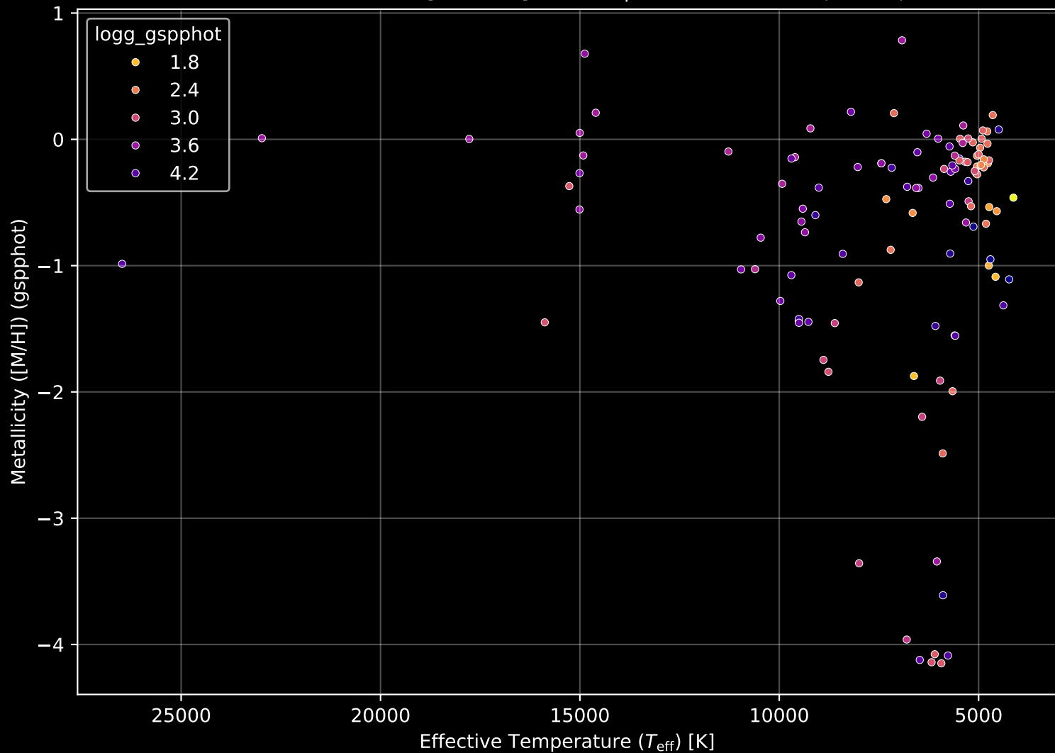
APOGEE DR17 Field: [288-00-C] Stellar Population Parameters (n= 119)
